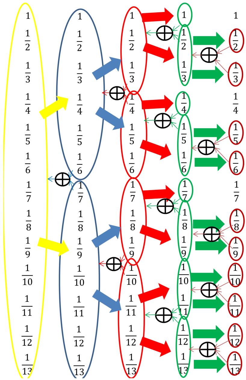
FIGURE 2 – Calcul récursif de H_{13} . L'algorithme est progressif - régressif. De gauche à droite, les données sont préparées, comme on organiserait le tableau d'un tournoi sportif. De droite à gauche, on en lit les résultats successifs. Ces derniers s'altèrent d'autant moins qu'ils sont appariés entre voisins de mêmes gabarits.
