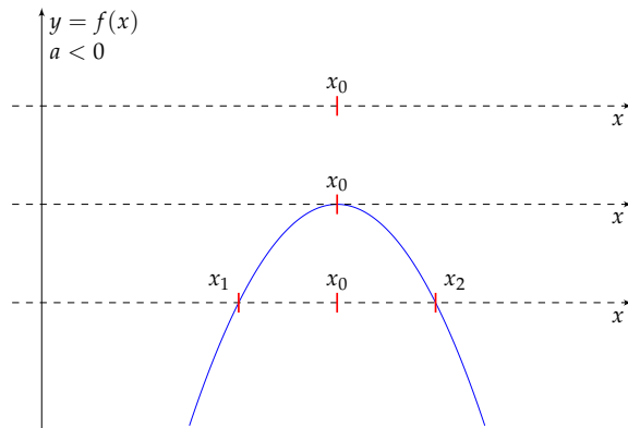
FIGURE 3 – Une grimace, c'est négatif! a < 0 . Trois positions sont ici représentées, selon que la parabole traverse, tangente ou évite l'axe des abscisses (qui apparaît en pointillés).
