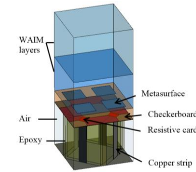
Fig. 1: Unit cell « egg-crate » type
