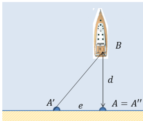
Figure 18 : Calcul de la distance (rectiligne) d'un navire à la côte avec deux amers.
