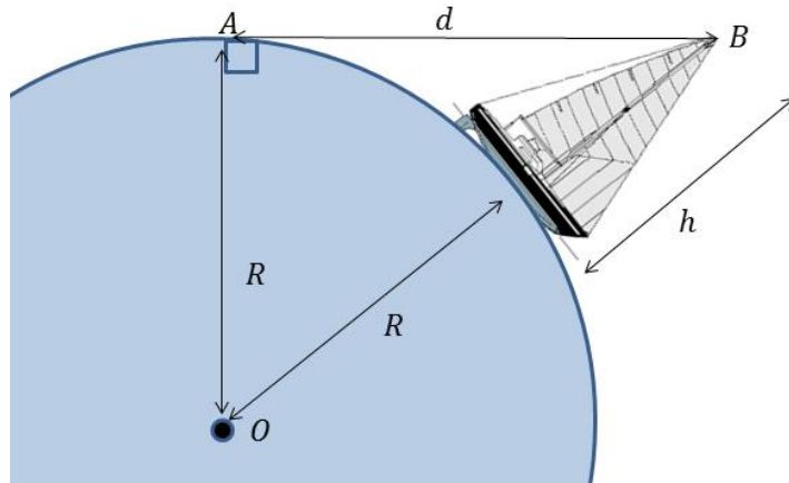
Figure 17 : La Terre emporte un voilier dans sa courbure (la figure n'est pas à l'échelle).
