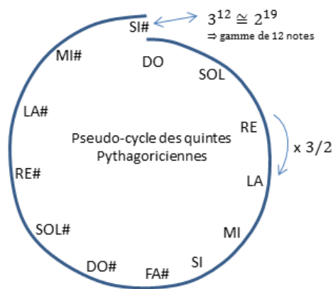
Figure 1 : spirale de quintes et gamme de Pythagore.
