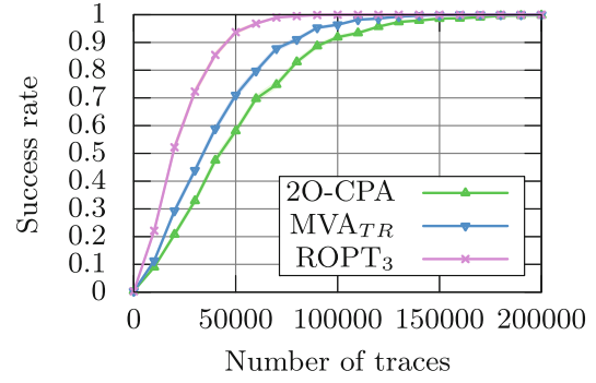
(d) \sigma = 7
