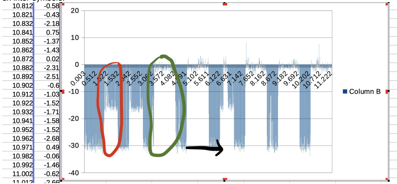
Fig 3), on peut en déduire les intervalles de valeur de champ magnétique pour un « 1 », pour un « 0 » et pour un inter-symbole.
