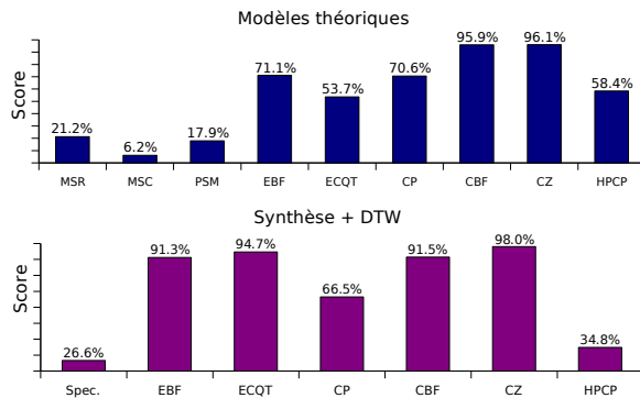
FIG. 3 – Résultats des différents systèmes testés sur la base de musique monophonique.
