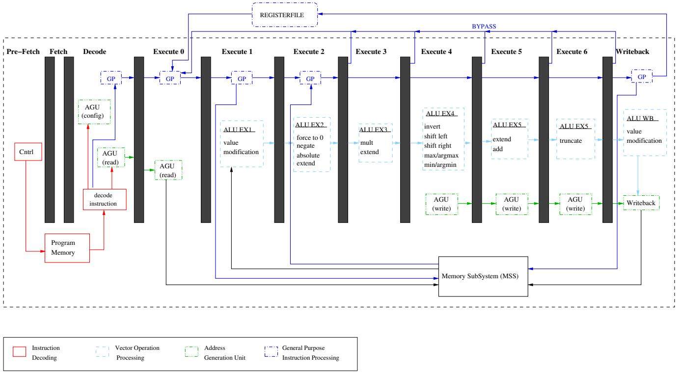
Fig. 3. ASIP Pipeline
