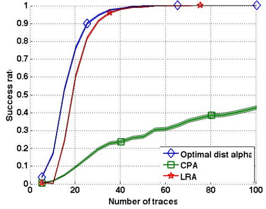
(d) \sigma_\alpha = 4, \sigma = 3
