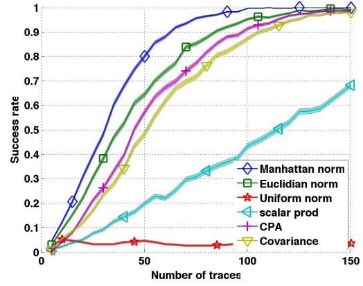
(d) Laplacian Noise, \sigma = 3
